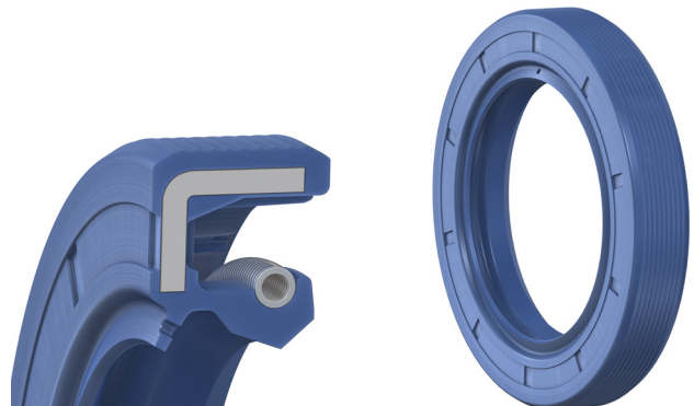
Abb. 1 BAUMSL mit entlüfteter Schutzlippe
