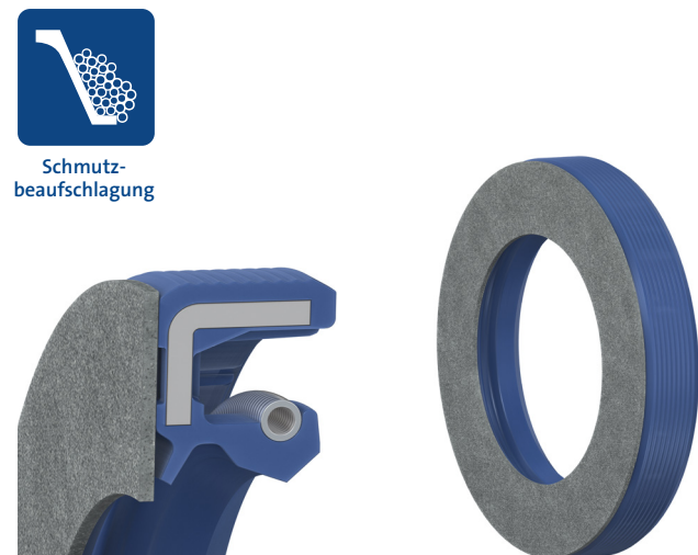
Abb. 4 BAUMSL kombiniert mit Vliesscheibe – für externe Schmutzbeaufschlagung
