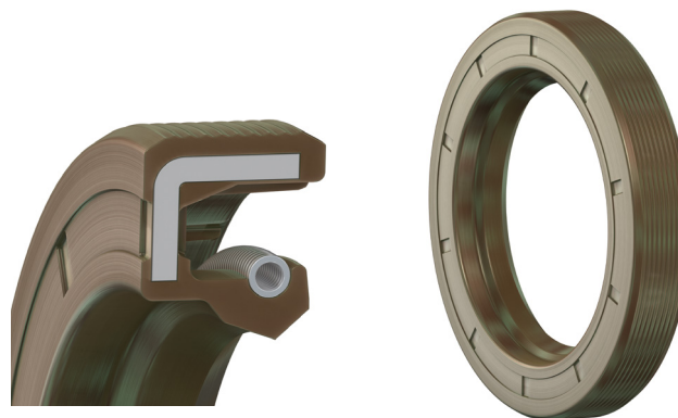
Abb. 8 Simmerring® Radial-Wellendichtring mit FKM PLUS-Coating
