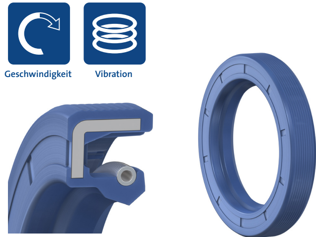
Abb. 3 Simmerring® Radial-Wellendichtring mit verstärkter Feder
