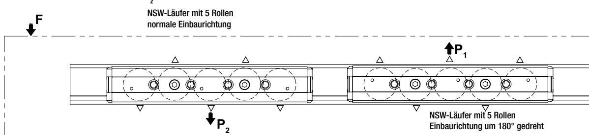
NSW-Läufer unter Lastmoment M_z
